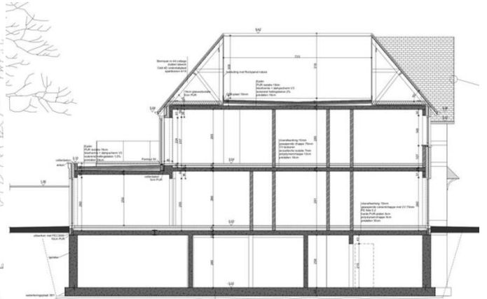
DOORSNEDE B - 1/50
