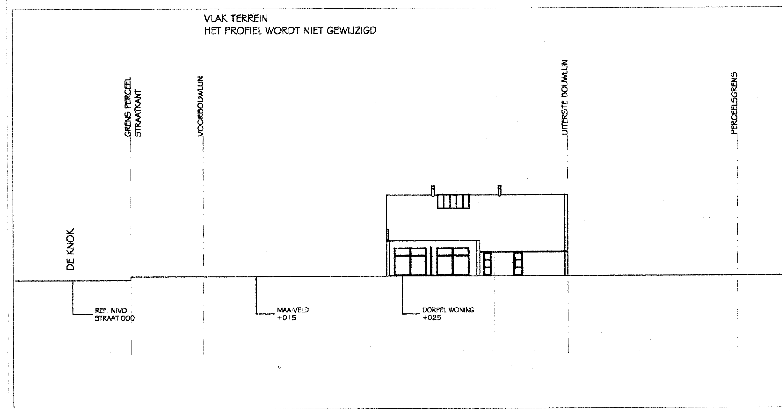
TERREINPROFIEL 1/250
